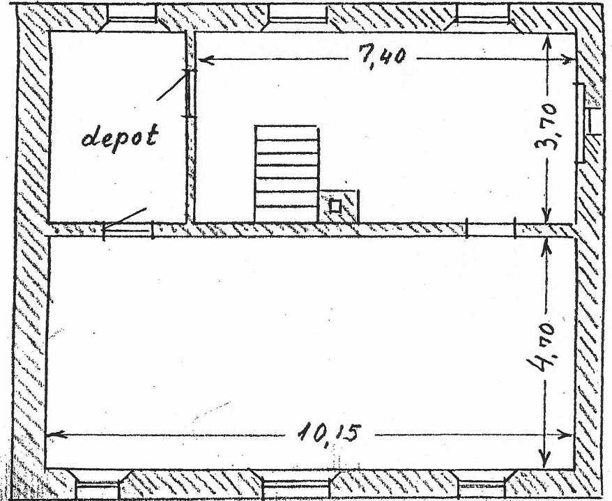
1. sal (1. floor)
